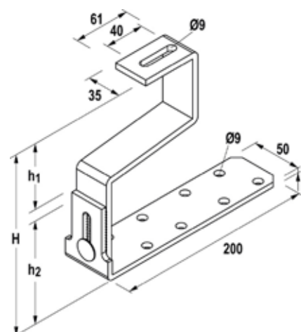
Állítható horog mediterrán cseréphez GC A2
