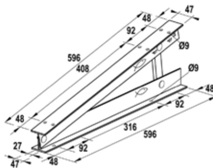
Előszerelt háromszög konzol STFS 10° - 13°
