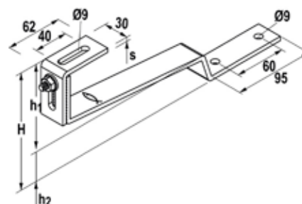
Állítható horog lapos cseréphez GTPR A2
