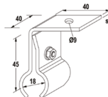
Csatlakozó állókorcos tetőhöz DLAK A2
