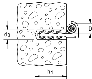
Clip fix plus egyes szorítókapocs SF plus ES
