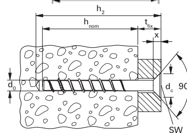
Betoncsavar FBS-US A4 - sülyesztett fejű, korrózióálló acél A4
