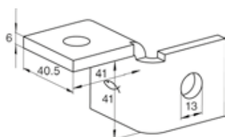
FUF 180°L hdg.
