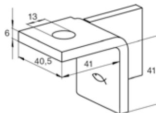
FUF 180°R hdg.
