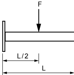
Terhelési eset 1
