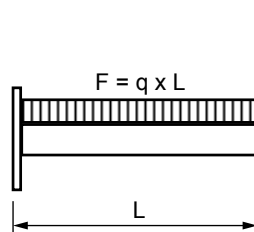
Terhelési eset 3
