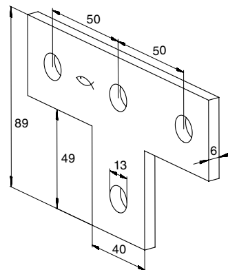
FFF 4T hdg.
