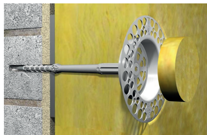
Felületbe süllyesztett rögzítés lágy szigetelőanyagok esetén
