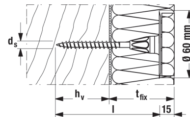
Sülyesztett szerelés
