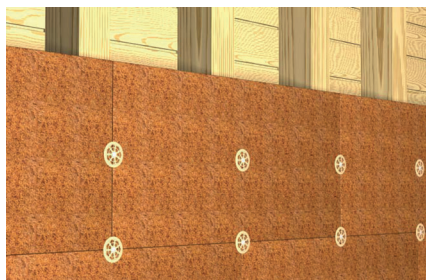
Faszálas táblák rögzítése tömör fánál
