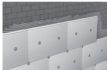
Polisztirol szigetelőtábla rögzítése üreges mészhomok téglára
